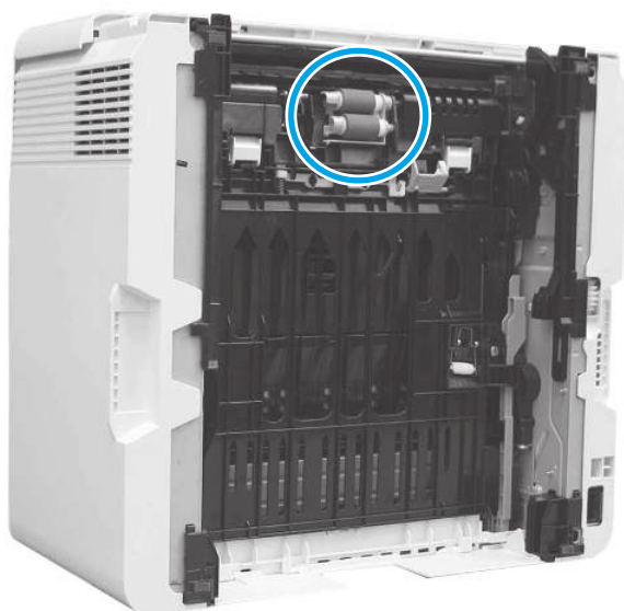
Figura 9-17 Limpieza de los rodillos
